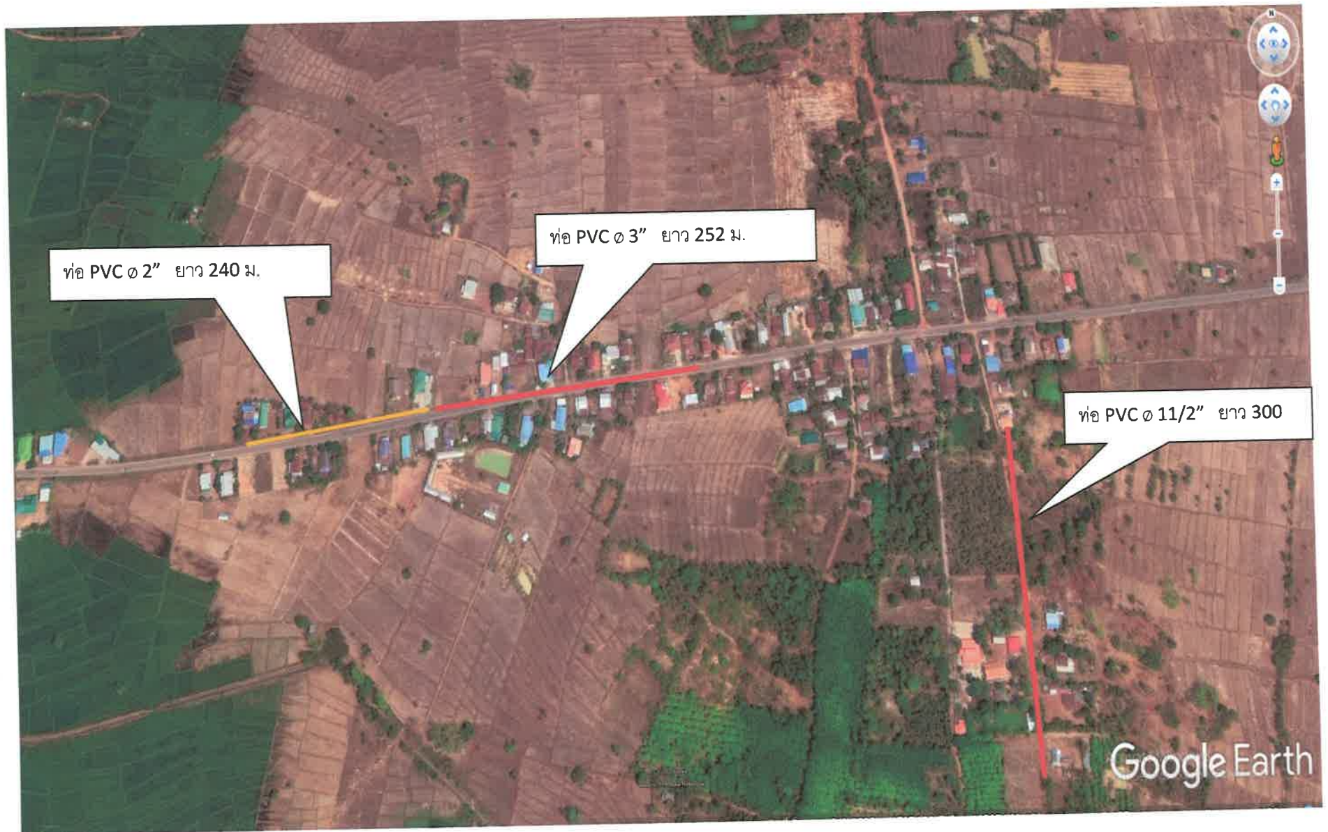
ขยายเขตประปาโดยวางท่อ PVC ๑ 3" ๑ 2 " และ 1 1/2" ยาว 792 เมตร หมู่ที่ 15 บ้านโนนภูทอง ตำบลเหล่าต่างคำ อำเภอโพธิ์ชัย จังหวัดหนองคาย
