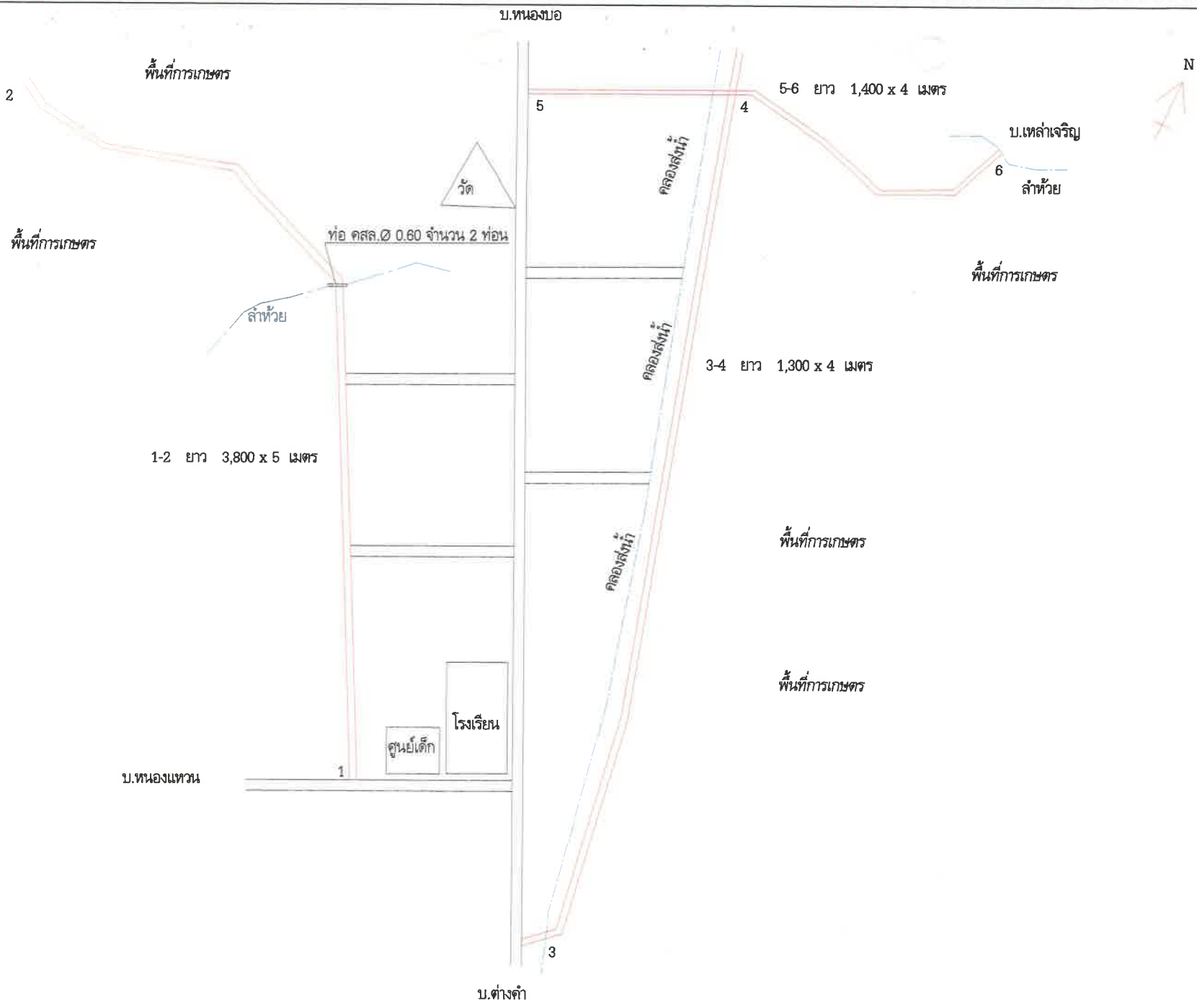
ผังสังเขปปรับปรุงซ่อมแซมถนนลูกรังสู่พื้นที่การเกษตร หมู่ที่ 3 ต.เหล่าต่างคำ อ.โพธิ์ชัย จ.หนองคาย
