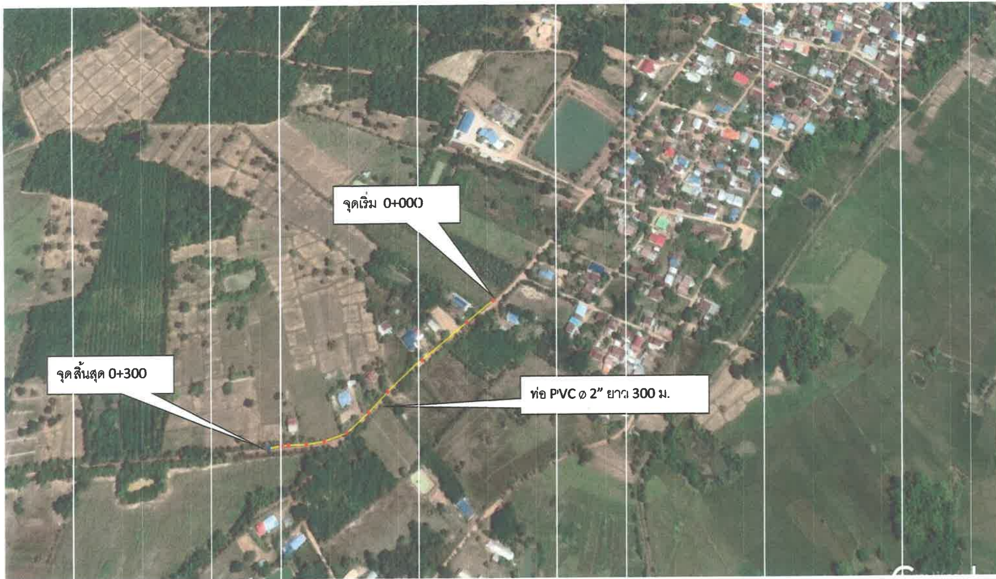
ขยายเขตประปาโดยวางท่อ PVC Ø 2" ยาว 300 เมตร หมู่ที่ 1 บ้านเหล่าต่างคำ ตำบลเหล่าต่างคำ อำเภอโพธิ์ชัย จังหวัดหนองคาย
